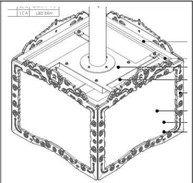
사각유리등 설계도 참고 예시
